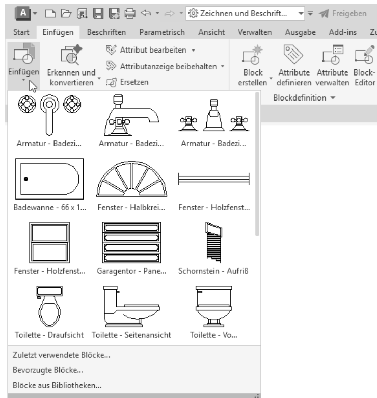
Galerie Blöcke
