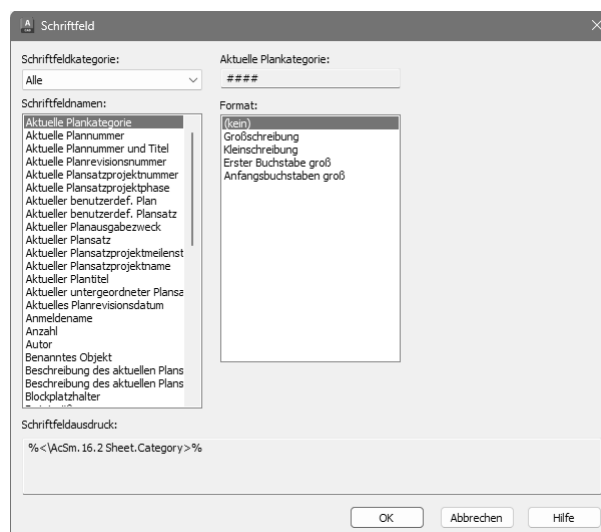
Dialog Schriftfeld
