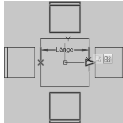
Aktion ANORDNEN
